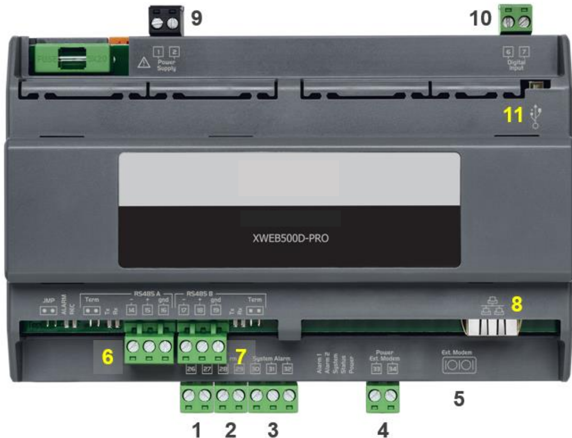
KLEMMLEISTE
